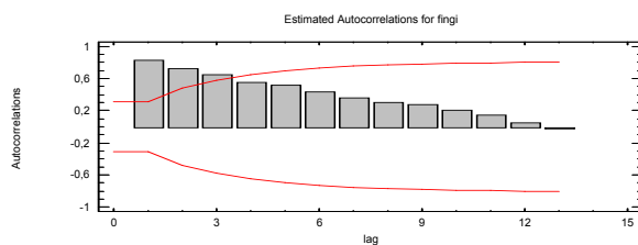
شكل بياني رقم (٢): رسم بياني لاستهلاك وتقديرات الارتباط الذاتي للفطرية في جمهورية مصر العربية.
