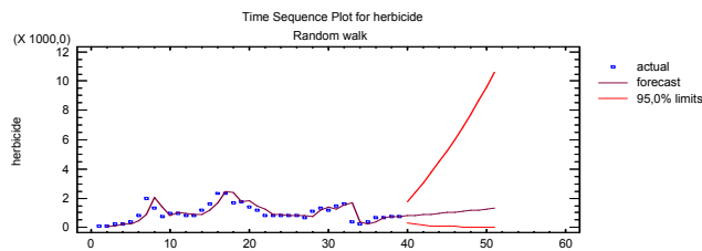
شكل بياني رقم (٧): رسم بياني للنماذج المختارة لاستهلاك مبيدات الحشائش في جمهورية مصر العربية. البيانات الحقيقية للفترة من ١٩٧٠-٢٠٠٨
