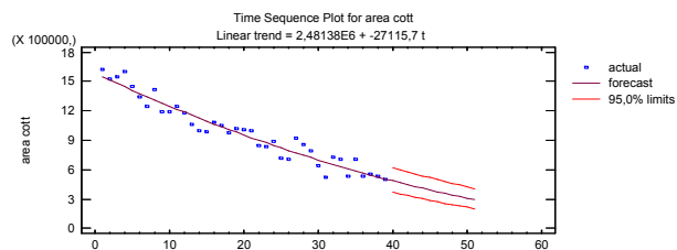
شكل بياني رقم (٨): رسم بياني للنماذج المختارة لمساحات محصول القطن في جمهورية مصر العربية.
