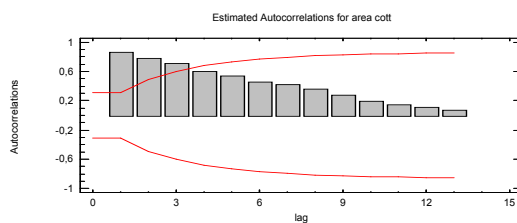
شكل بياني رقم (٤): رسم بياني لمساحات وتقديرات الارتباط الذاتي لمحصول القطن في جمهورية مصر العربية.
