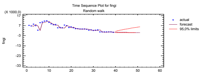
شكل بياني رقم (٦): رسم بياني للنماذج المختارة لاستهلاك المبيدات الفطرية في جمهورية مصر العربية.
