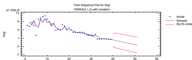
شكل بياني رقم (٥): رسم بياني للنماذج المختارة لاستهلاك المبيدات الحشرية في جمهورية مصر العربية. البيانات الحقيقية للفترة من ١٩٧٠-٢٠٠٨
