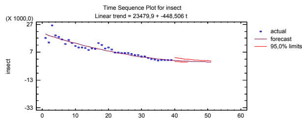
شكل بياني رقم (٥): رسم بياني للنماذج المختارة لاستهلاك المبيدات الحشرية في جمهورية مصر العربية. البيانات الحقيقية للفترة من ١٩٧٠-٢٠٠٨
