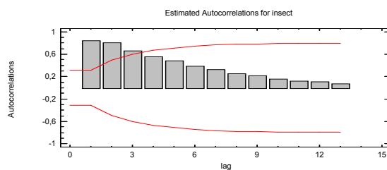
شكل بياني رقم (١): رسم بياني لاستهلاك وتقديرات الارتباط الذاتي للمبيدات الحشرية في جمهورية مصر العربية.
