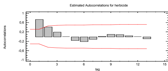
شكل بياني رقم (٣): رسم بياني لاستهلاك و تقديرات الارتباط الذاتي لمبيدات الحشائش في جمهورية مصر العربية.
